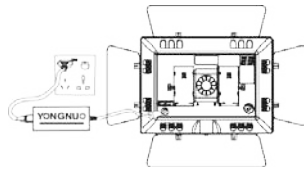
Можно подключить источник постоянного тока (19 В, 5 А)
