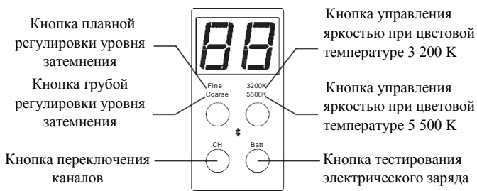
Управляющие кнопки для осветителя YN900 с двумя цветными фильтрами
