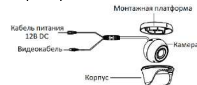
Рисунок 1-14 Камера «шар» I типа
