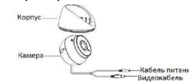
Рисунок 1-16 Камера «шар» II типа
