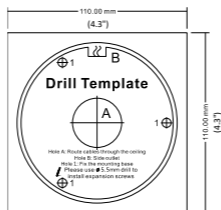
Рисунок 2-2 Шаблон крепления
